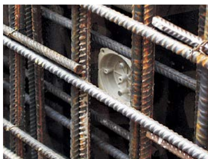
A zsaluzatra erősített KBV fedél.
