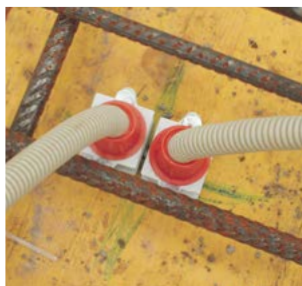
A végelem és a kivezető alkalmazásának példája.
