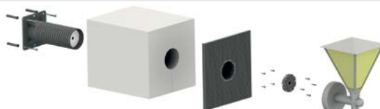
MDZ XL, MDZ XL 300 - szerelőlemez hőszigetelő burkolatba
