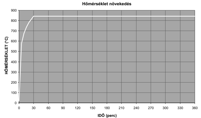
A hőmérséklet növekedése a vizsgálati kemence felmelegítése során, az egységesített hőmérsékleti görbe (ETK) szerint
